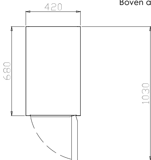
Boven aanzicht
